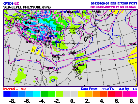
圖 4 A 為實驗 1 (NODA_NOGWD) 預報 72 小時海平面氣壓 (藍線) 及 ECMWF 分析場 (紅線) 之月平均及兩者之差值 (以顏色表示)。B 同 A 圖, 但為實驗 2 (NODA_GWD1)。
