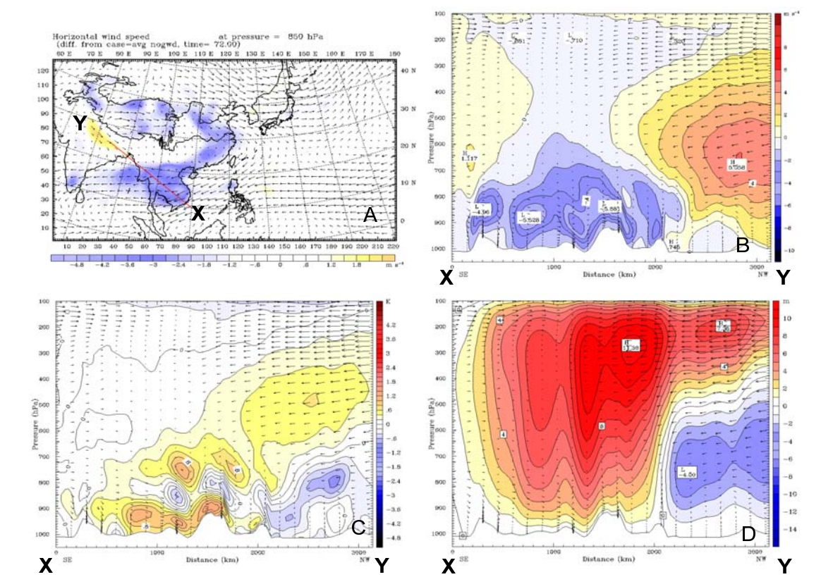
圖 8 A 為實驗 2 (NODA_GWD1) 與實驗 1 (NODA_NOGWD) 72 小時預報 850 hPa 風速之月平均差值場 (顏色分布)。B、C、D 為 A 圖中紅線之垂直剖面圖，其中 B 為風速差值場 (單位 m/s)，C 為溫度差值場 (單位 ^{\circ}\text{C} )，D 為重力位高差值場 (單位 m)。風標皆為實驗 2 之 72 小時預報風場。
