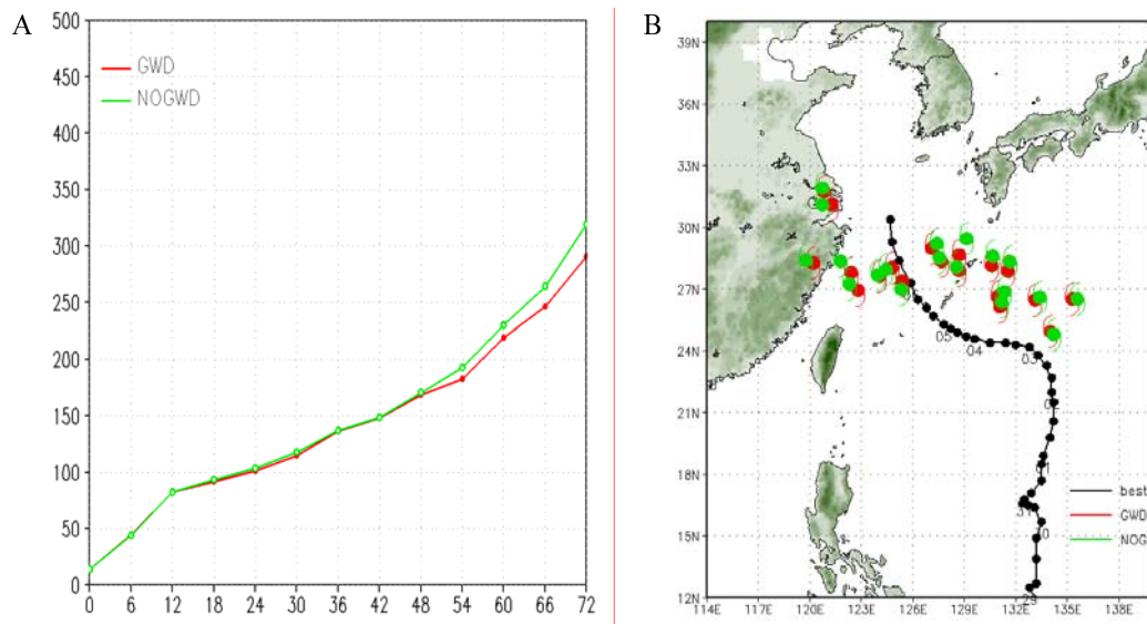
圖 9 A 為梅花 (Muifa) 颱風之平均路徑預報誤差，其中紅線為有使用 GWD 參數法之實驗 (UPD_GWD1)，綠線則為未使用 GWD 參數法之實驗 (UPD_NOGWD)。B 為梅花 (Muifa) 颱風之最佳路徑 (黑色點線) 以及 19 個 UPD_GWD1 實驗 (紅點) 和 UPD_NOGWD 實驗 (綠點) 預報第 72 小時之颱風位置。
