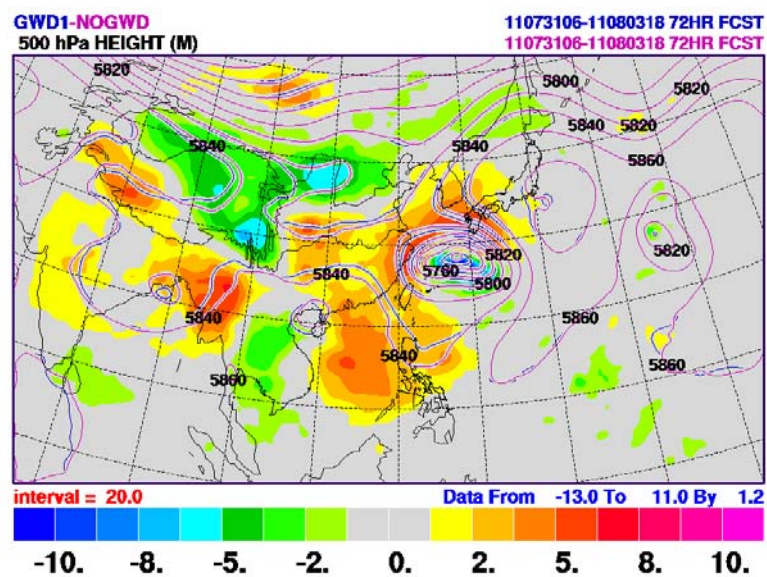
圖 10 梅花 (Muifa) 颱風預報實驗期間，72 小時預報之 500 hPa 高度場的合成圖，藍線為 UPD_GWD1 實驗，紫線為 UPD_NOGWD 實驗，兩個實驗之高度場預報的差值以顏色表示。
