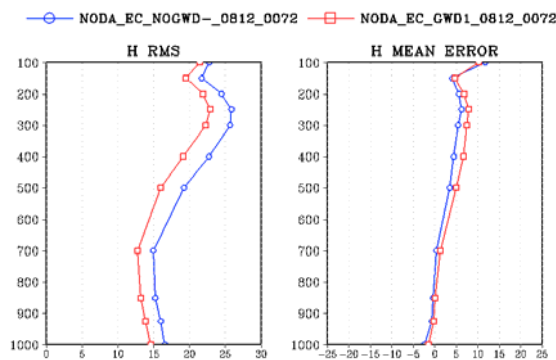
圖 2 實驗 1 (NODA_NOGWD, 藍線) 與實驗 2 (NODA_GWD1, 紅線) 之 72 小時預報對 ECMWF 分析場的校驗結果。A 為 U 分量 (單位 m/s) 之均方根誤差 (左) 和平均誤差 (右), B 為 V 分量 (單位 m/s), C 為重力位高度場 (單位 m), D 為溫度場 (單位 K)。
