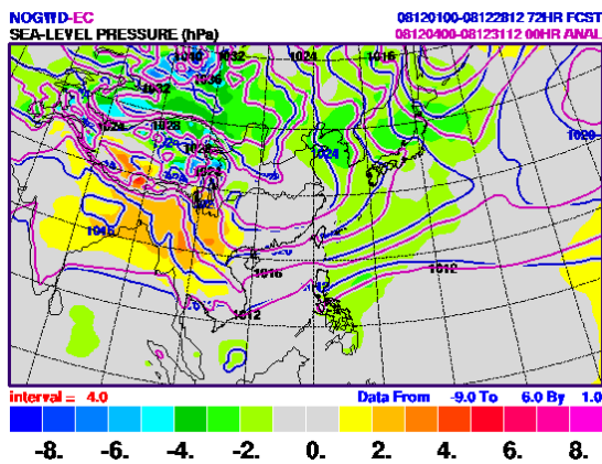
圖 4 A 為實驗 1 (NODA_NOGWD) 預報 72 小時海平面氣壓 (藍線) 及 ECMWF 分析場 (紅線) 之月平均及兩者之差值 (以顏色表示)。B 同 A 圖, 但為實驗 2 (NODA_GWD1)。
