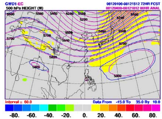
圖 3 A 為實驗 1 (NODA_NOGWD) 之預報 72 小時 500 hPa 溫度場 (藍線) 與 ECMWF 分析場 (紅線) 之月平均及兩者之差值 (以顏色表示)。B 圖同 A 圖, 但為實驗 2 (NODA_GWD1)。C 圖與 D 圖則為 500 hPa 重力位高度。
