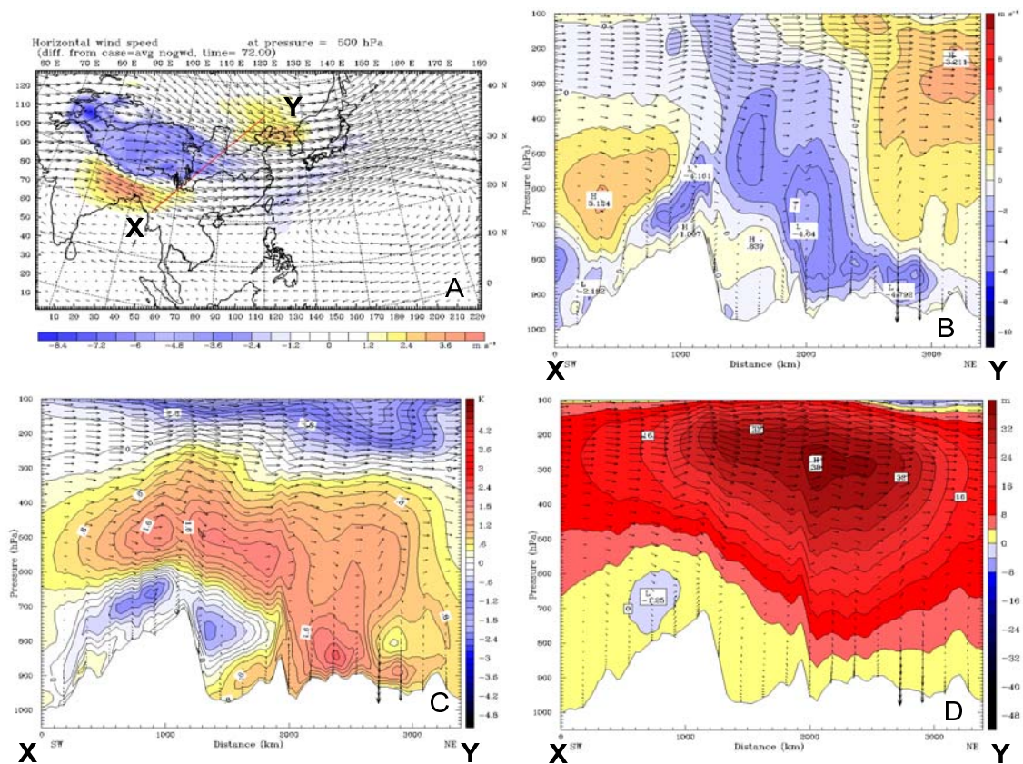
圖 7 A 為實驗 2 (NODA_GWD1) 與實驗 1 (NODA_NOGWD) 72 小時預報 500 hPa 風速之月平均差值場(顏色分布)。B、C、D 為 A 圖中紅線之垂直剖面圖,其中 B 為風速差值場(單位 m/s),C 為溫度差值場(單位 K),D 為重力位高差值場(單位 m)。風標皆為實驗 2 之 72 小時預報風場。
