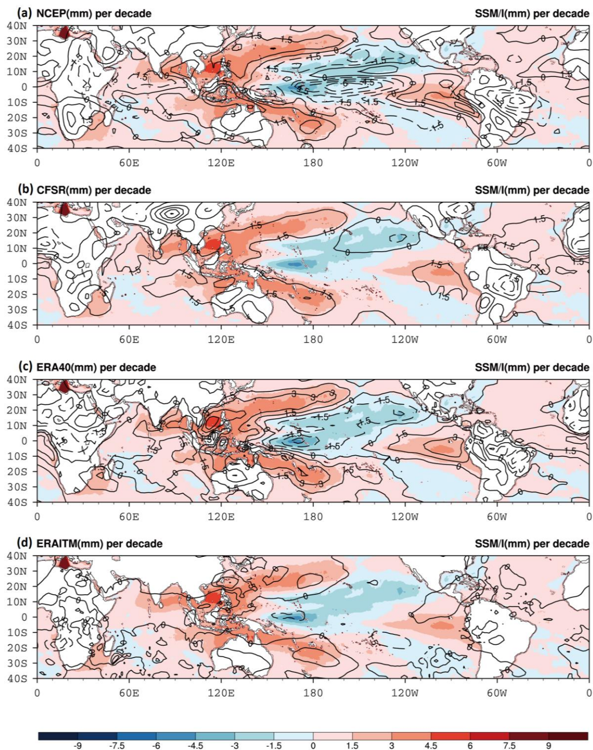
圖 2 (a) NCEP-R2, (b) CFSR, (c) ERA-40 以及(d) ERA-interim 垂直積分氣柱水汽量（等值線）和 SSM/I 反演氣柱水汽量（色階）的時間變化趨勢比較。資料時間取 1989~2001 年間之變化趨勢，單位為 \text{mm decade}^{-1} 。
