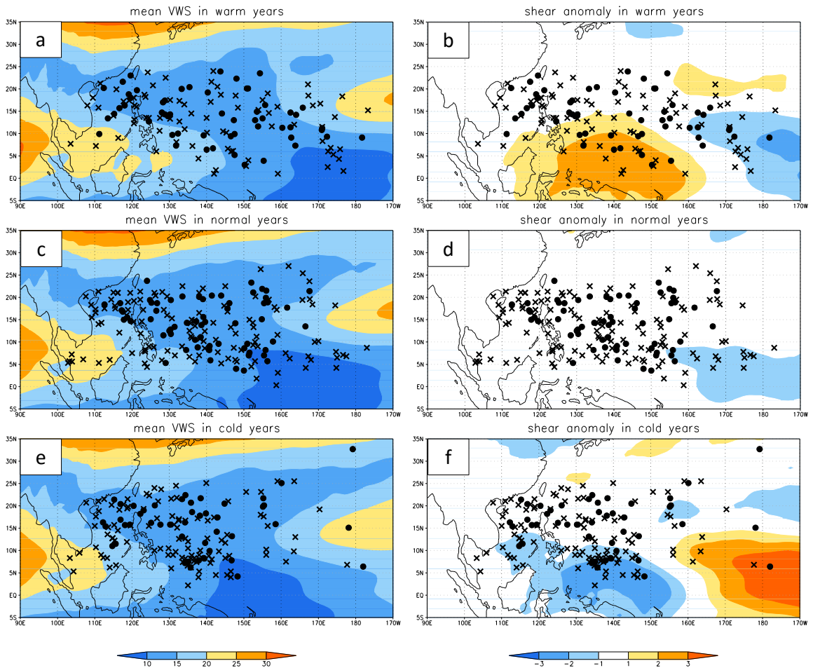
圖 4 同圖 1，但左邊為 200hPa-850hPa 垂直風切速度（色階，單位 \text{ms}^{-1} ），右邊為 200hPa-850hPa 垂直風切距平（色階，單位 \text{ms}^{-1} ）。黑點為 TCd，叉號為 TCn。
