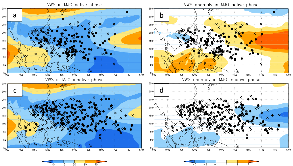
圖 14 同圖 11, 但左邊為 200\text{hPa} – 850\text{hPa} 垂直風切 (色階, 單位 \text{ms}^{-1} )。右邊為 200\text{hPa} – 850\text{hPa} 垂直風切距平 (色階, 單位 \text{ms}^{-1} )。黑點為 TCd, 叉號為 TCn。
