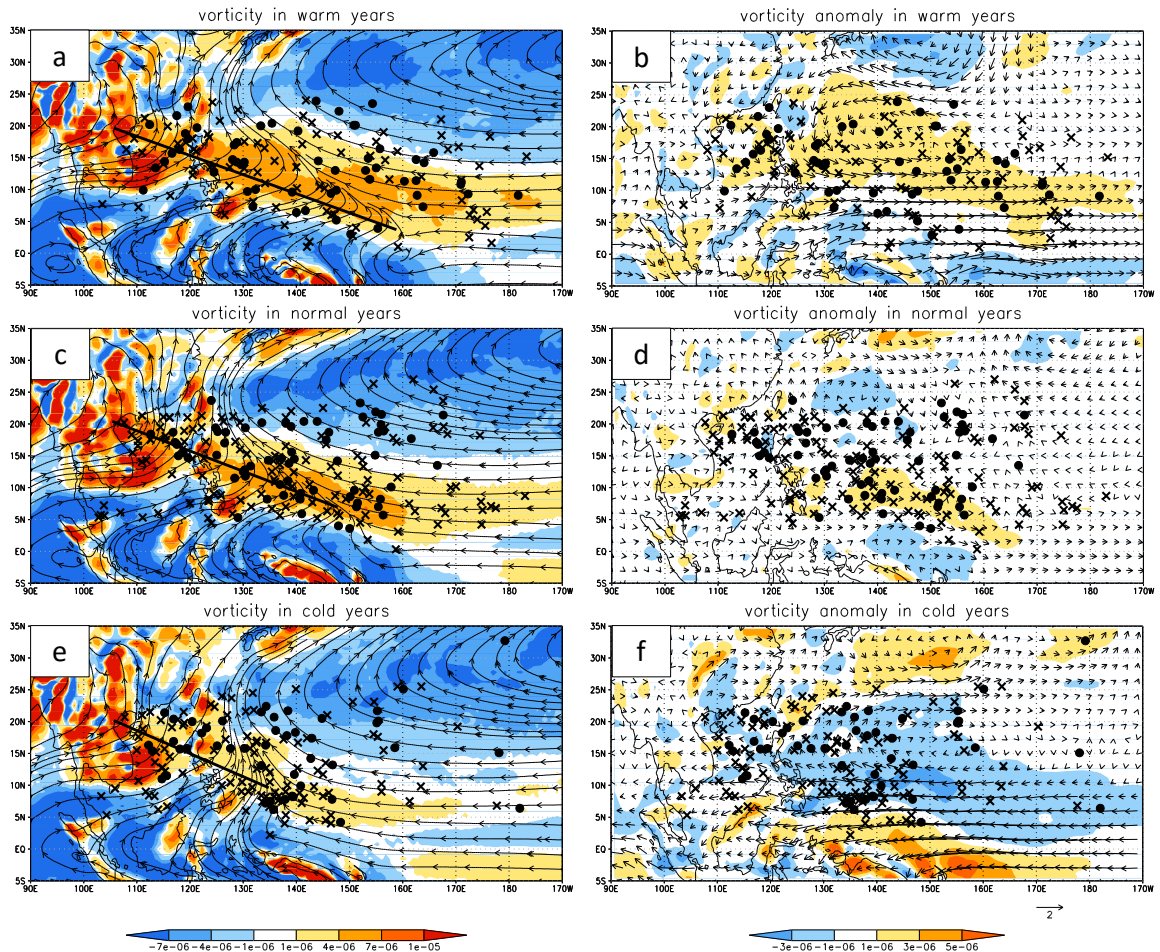
圖 2 同圖 1，但左邊為 850hPa 相對渦度 (色階，單位 \text{s}^{-1} ) 與流線場，黑色實線概略表示季風槽軸。右邊為 850hPa 渦度距平 (色階，單位 \text{s}^{-1} ) 與風場距平 (單位 \text{ms}^{-1} )。黑點為 TCd，叉號為 TCn。
